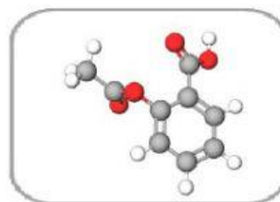
Slika 3: Slika krogličnega modela molekule acetilsalicilne kisline (povezava do interakt. prikaza)
