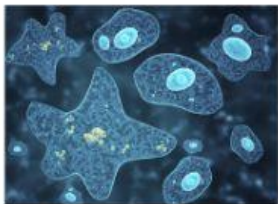
Amebes
