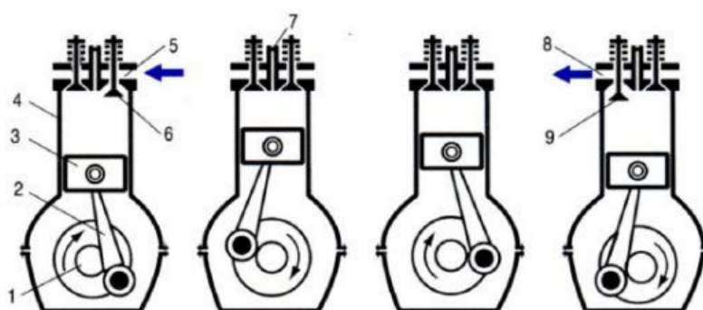
Hình 21.2: Sơ đồ chu trình làm việc của động cơ điêzen 4 kì
