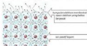
Gambar ikatan logam
