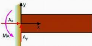
Menahan Momen, Gaya Horizontal, dan Gaya Vertikal
