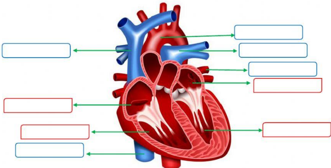
Gambar 1. Bagian-bagian Jantung
