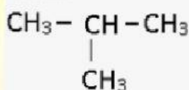
2-metilpropana
