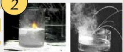
Gambar 4. Reaksi logam natrium dengan air (Sumber: m-edukasi.kemendikbud.go.id)
