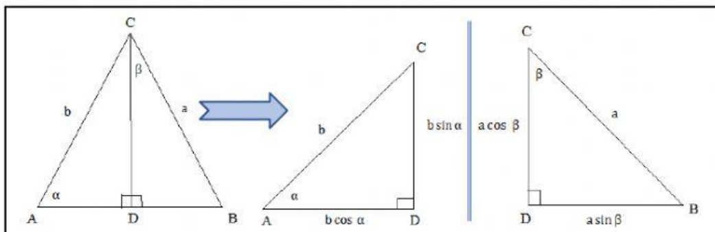
Gambar 1.2. Segitiga ABC
