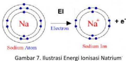
Gambar 7. Ilustrasi Energi Ionisasi Natrium
