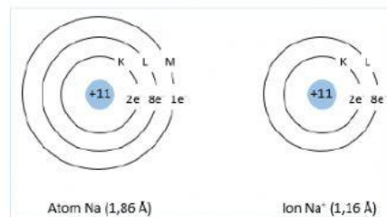
Gambar 5. Ilustrasi Jari-jari atom _{11}\text{Na} dan jari-jari ion _{11}\text{Na}^+
