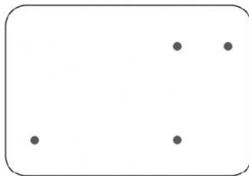
triangolo ottusangolo
