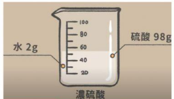
硫 酸
