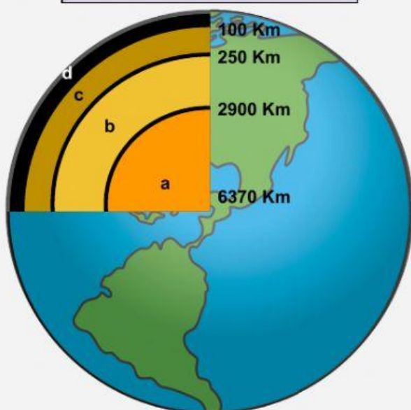
MODEL GEODINÀMIC
