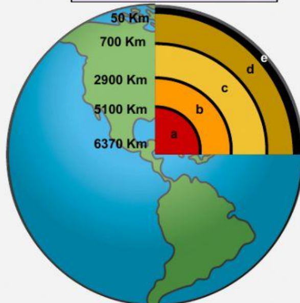
MODEL GEOQUÍMIC
