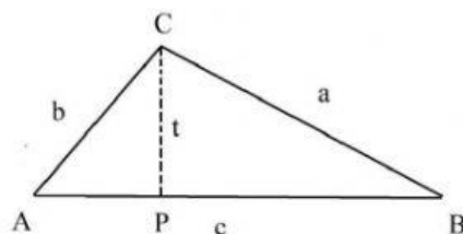
Gambar (1) Segitiga ABC
