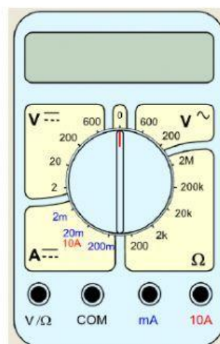
Mesure d'une résistance d'environ 500 Ω
