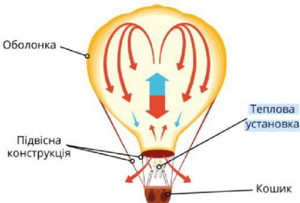
Будова аеростата
