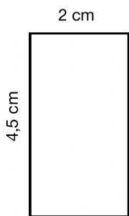
paral·lelogram (rectangle)
