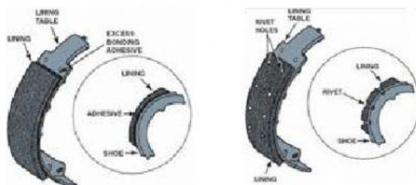
Gambar 1. 9 Sepatu rem
