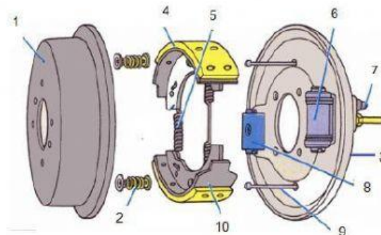
Gambar 1. 3 Komponen rem tromol
