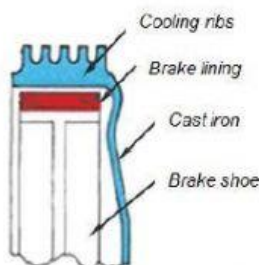
Gambar 1. 5 Penampang tromol dari besi cor
