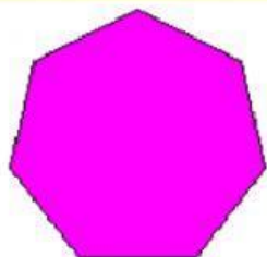
HEPTÁGONO REGULAR
