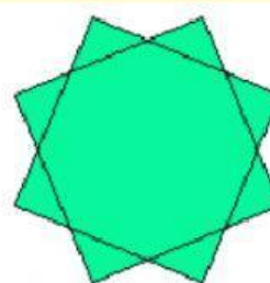
OCTÓGONO ESTRELLADO
