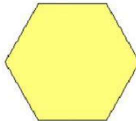
HEXÁGONO REGULAR
