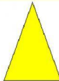
TRIÁNGULO ISÓSCELES
