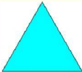
TRIÁNGULO EQUILÁTERO
