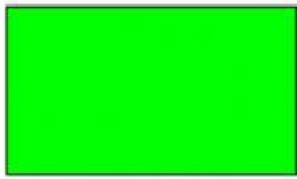
RECTÁNGULO
