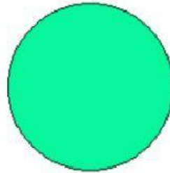
CÍRCULO
