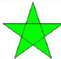
PENTÁGONO ESTRELLADO
