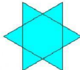
HEXÁGONO ESTRELLADO
