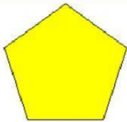
PENTÁGONO REGULAR
