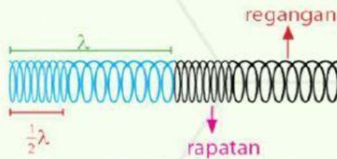
Gambar 2. Gelombang longitudinal
