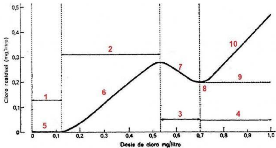
Curva generalizada, obtenida durante la cloración al break-point
