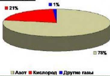
Состав воздуха
