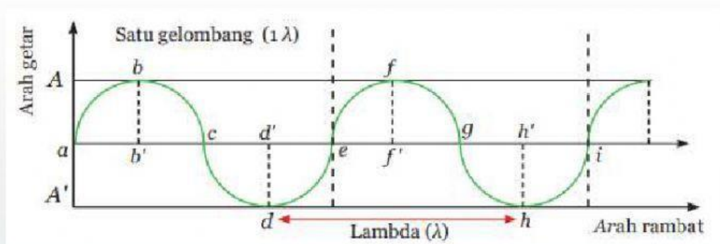
Sumber : Dok. Kemendikbud Gambar 1. Gelombang Transversal
