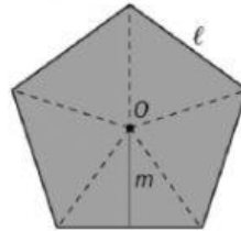
■ Pentágono regular.
