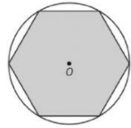
■ Hexágono inscrito.
