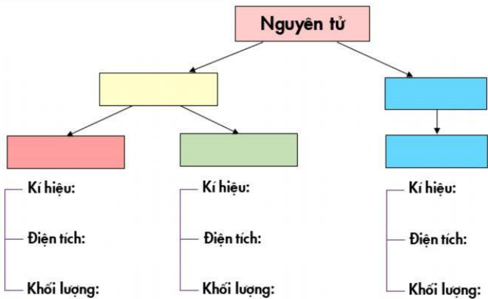
Hình 2.2. Sơ đồ tổng kết cấu tạo nguyên tử.
