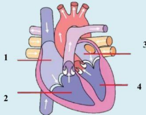
Gambar 1 Bagian Jantung
