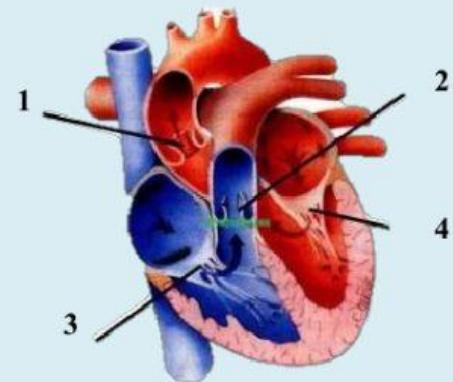
Gambar 2 Katup Jantung
