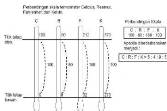
Gambar 10 Perbandingan skala termometer Sumber:
