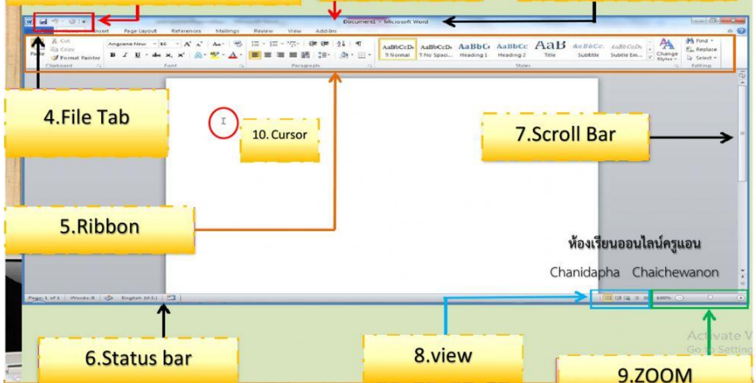
2.Title Bar
