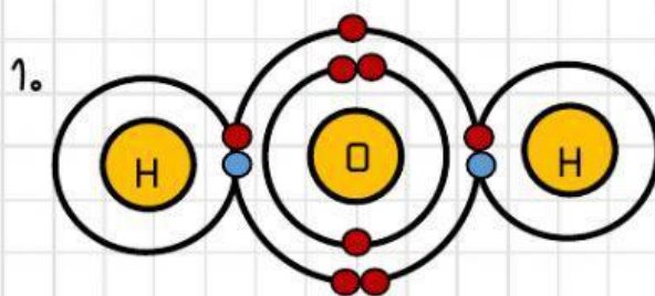
สูตรโมเลกุลของน้ำ (H 2 O)
