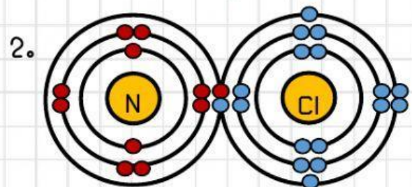
สูตรโมเลกุลของเกลือ (NaCl)
