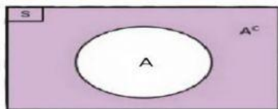
Diagram Venn A^c
