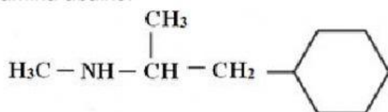
N-metil-2-cicloexil-1-metiletanamina
