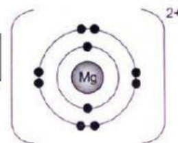
Ion magnesium (2.8) Magnesium ion (2.8)
