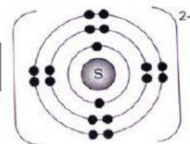
Ion sulfida (2.8.8) Sulphide ion (2.8.8)
