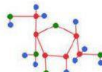
Estructura del anillo de fructosa
